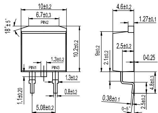
TO-263(D 2 PAK) MUR10XXB
