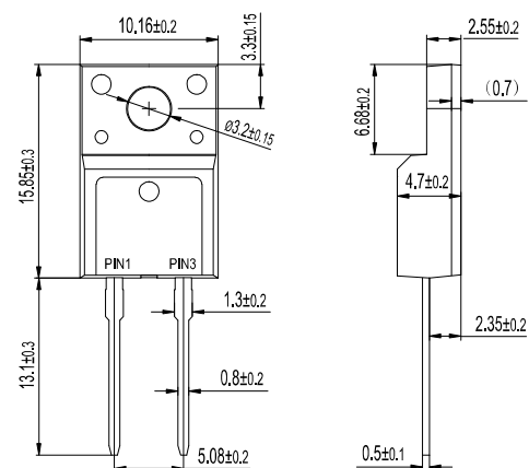
ITO-220AC MUR10XXF
